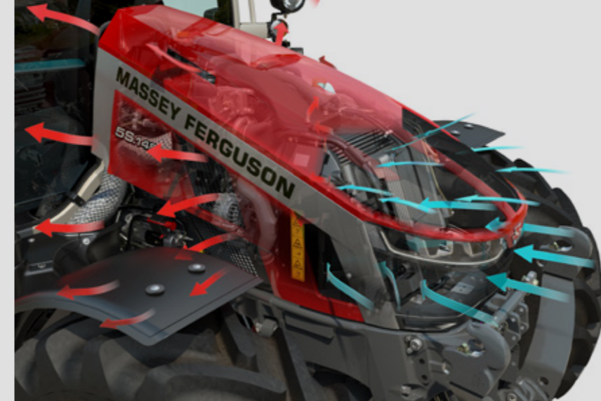
Ein neues, optimiertes Luftführungssystem verbessert die Motorkühlung und steigert sowohl Leistungsfähigkeit als auch Effizienz. Dank des neuen Designs der Belüftungsschlitze werden alle Kühler maximal und effizient mit Frischluft durchströmt.
