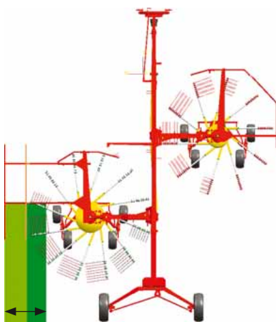
EUROTOP 651 A
