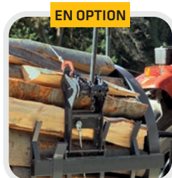
Cliquet tendeur.
