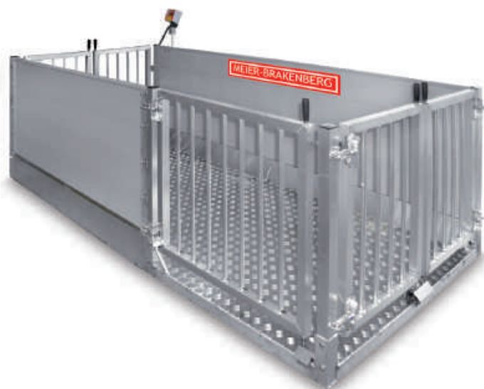
Stationäre Waage mit zusätzlichem Seitentor
