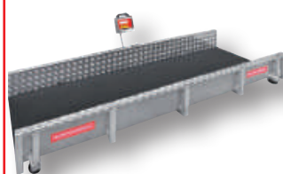
Pferdewaage mit gummiertem Boden für Tierklinik
