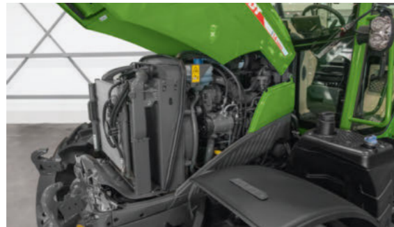
Der Motorraum ist zur Kontrolle und Wartung sehr einfach zugänglich, auch mit Frontladerbauteilen. Die Haube mit zwei separaten Seitenteilen ist komfortabel zu öffnen.
