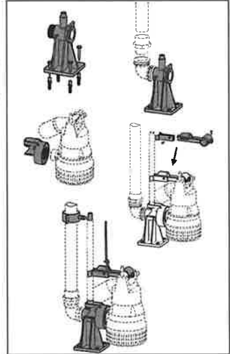
Einbaubeispiel / Installation example
