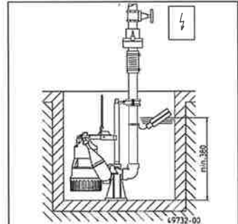
Einbaubeispiel / Installation example
